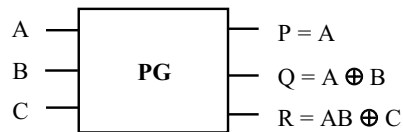
Fig.3. Peres Gate
