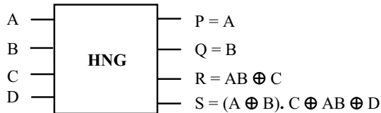
Fig.4. Haghparast Navi Gate
